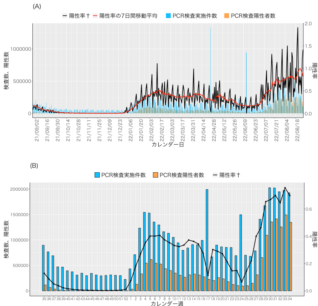
図 2: PCR 検査数、PCR 陽性者数、陽性率 † : (A)日別、(B)週別(2021 年 8 月 30 日~2022 年 8 月 29 日)
